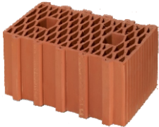
38 Petek İzo Tuğla (W Sınıfı)
